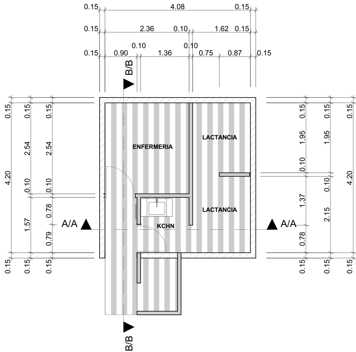
PLANTA DIMENSIONADA ESC.: 1:50
