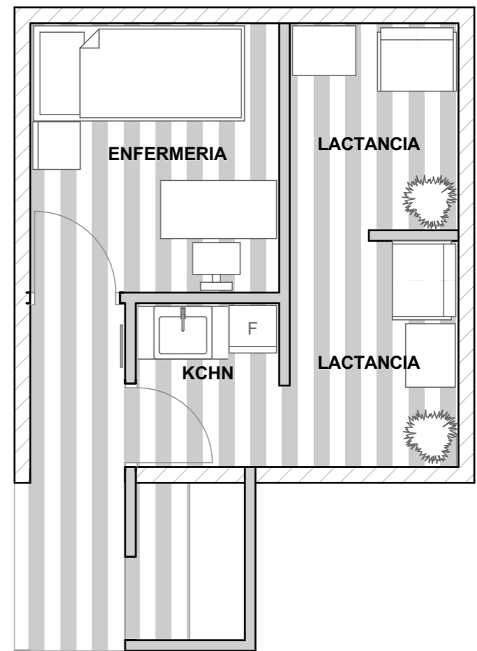
PLANTA ARQUITECTONICA ESC.: 1:50
